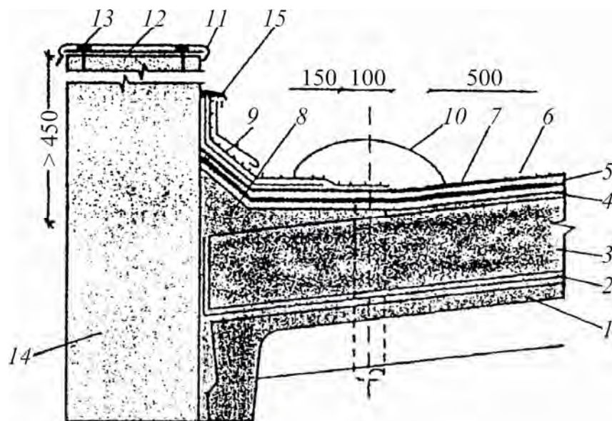
Рис. 33. Примыкание кровли к парапету высотой более 450 мм: 1 — сборная железобетонная плита покрытия; 2 — пароизоляция (по расчету); 3 — теплоизоляция; 4 — выравнивающая стяжка; 5 — нижний слой основного кровельного ковра; 6 — верхний слой основного кровельного ковра; 7 — крупнозернистая посыпка; 8 — наклонный бортик; 9 — слои дополнительного кровельного ковра; 10 — воронка внутреннего водостока; 11 — оцинкованная кровельная сталь; 12 — костыли 40 × 4 через 600 мм; 13 — дюбели; 14 — стена; 15 — герметизирующая мастика
