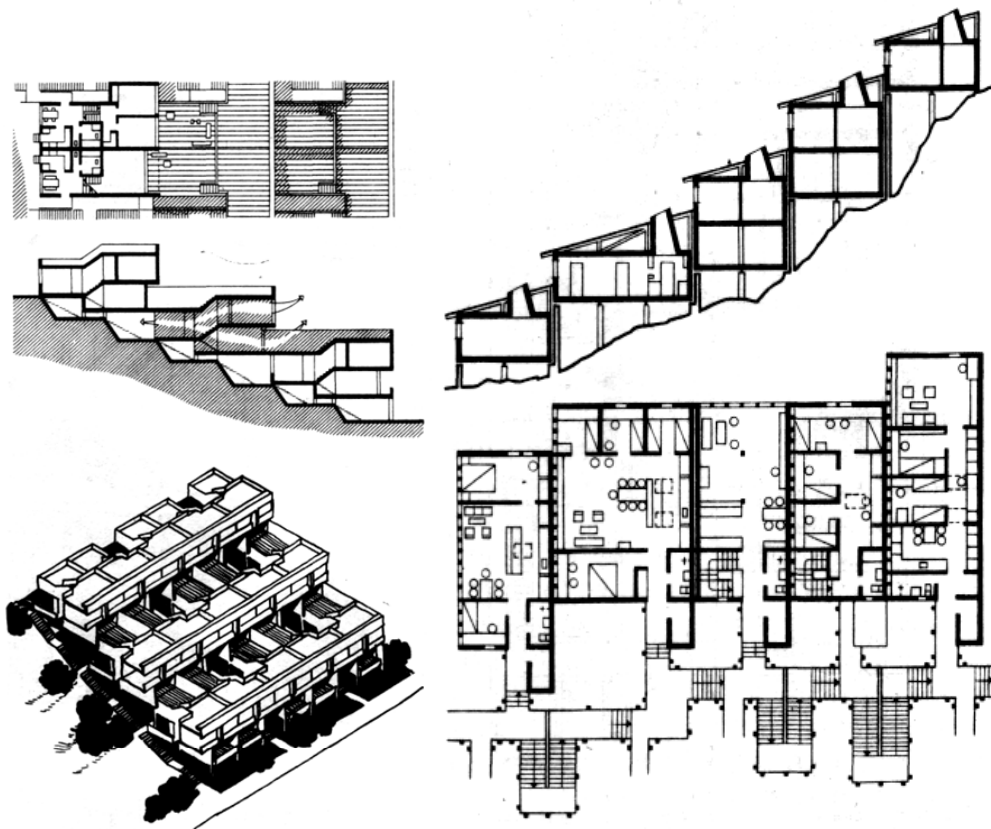
Рис. 51. Террасные блокированные дома на участках с сильным рельефом: слева — жилой дом с блоками прямоугольной формы, расположенными поперек рельефа (Швейцария); справа — жилые дома с прямоугольными одно-, двухэтажными блоками, расположенными вдоль рельефа (Гренландия)
