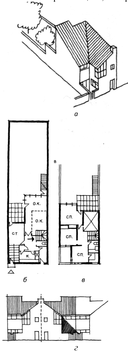
Рис. 36. Четырехкомнатная двухэтажная блок-квартира с двухсветной общей комнатой: а — общий вид блок - квартиры; б — план первого этажа; в — план второго этажа; г — фасад дома
