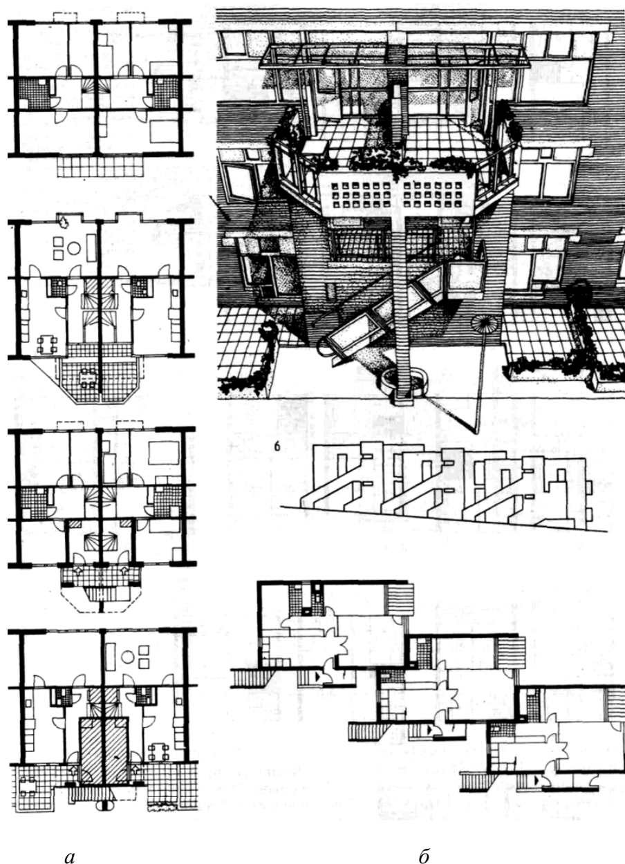
Рис. 33. Блокированные дома с поэтажными квартирами и с входами с наружных лестниц: а — четырехэтажный дом с двухэтажными квартирами (Голландия), б — двухэтажный дом (Венгрия): фасад, планы этажей
