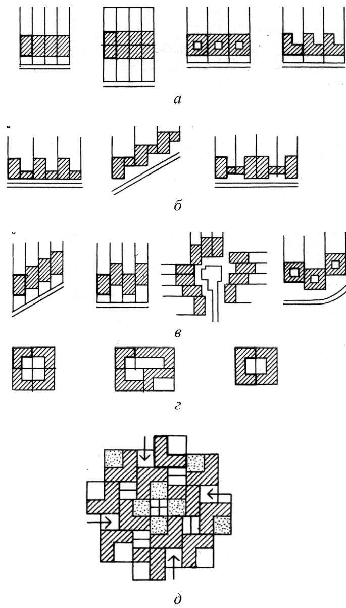
Рис. 54. Приемы блокировки блок – квартир: а — линейная; б — со сдвигом; в — через хозяйственные пристройки; г — с образованием замкнутых двориков; д — сплошная (ковровая) застройка
