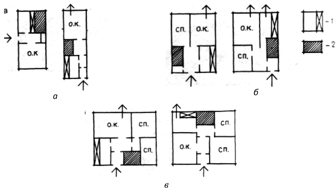
Рис. 31. Схемы построения одноэтажных блок-квартир:
