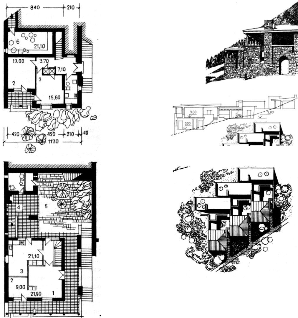
Рис. 53. Высокогорное село Гудани (Грузия). Пример террасной застройки в сельском строительстве. Общий вид, план первого этажа, план второго этажа, генеральный план, разрез: 1 — общая комната; 2 — спальни; 3 — кухня-столовая; 4 — летняя кухня; 5 — внутренний дворик; 6 — подвал
