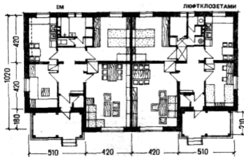
Рис. 22. Двухквартирный одноэтажный дом с вариантами инженерного оборудования. Фасад, план этажа
