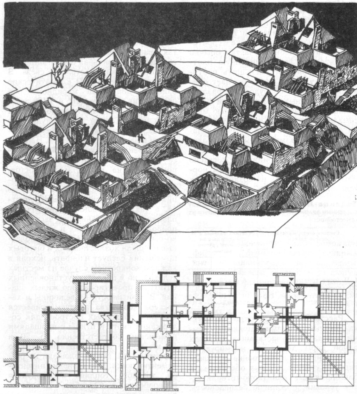
Рис. 57. Жилой квартал в Горисе (Армения), архитекторы Г. Погосян, А. Мкртчак, Г. Согоян. Жилые дома расположены на рельефе. В каждом доме в зависимости от рельефа семь или восемь квартир с самостоятельным входом с улицы и широкая терраса. Общий вид (рисунок с макета), планы этажей
