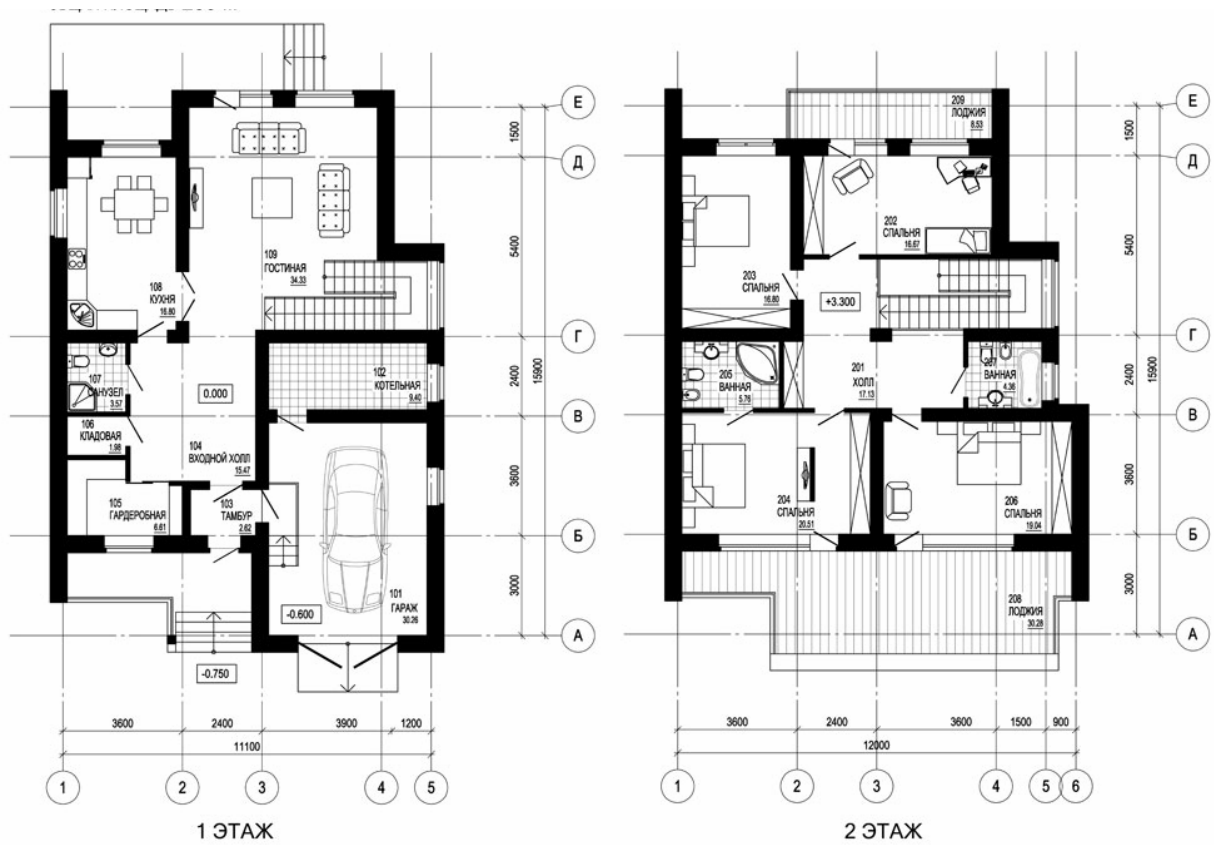
Рис. П.54. Общие виды двухэтажного жилого дома. Вариант «Т»
