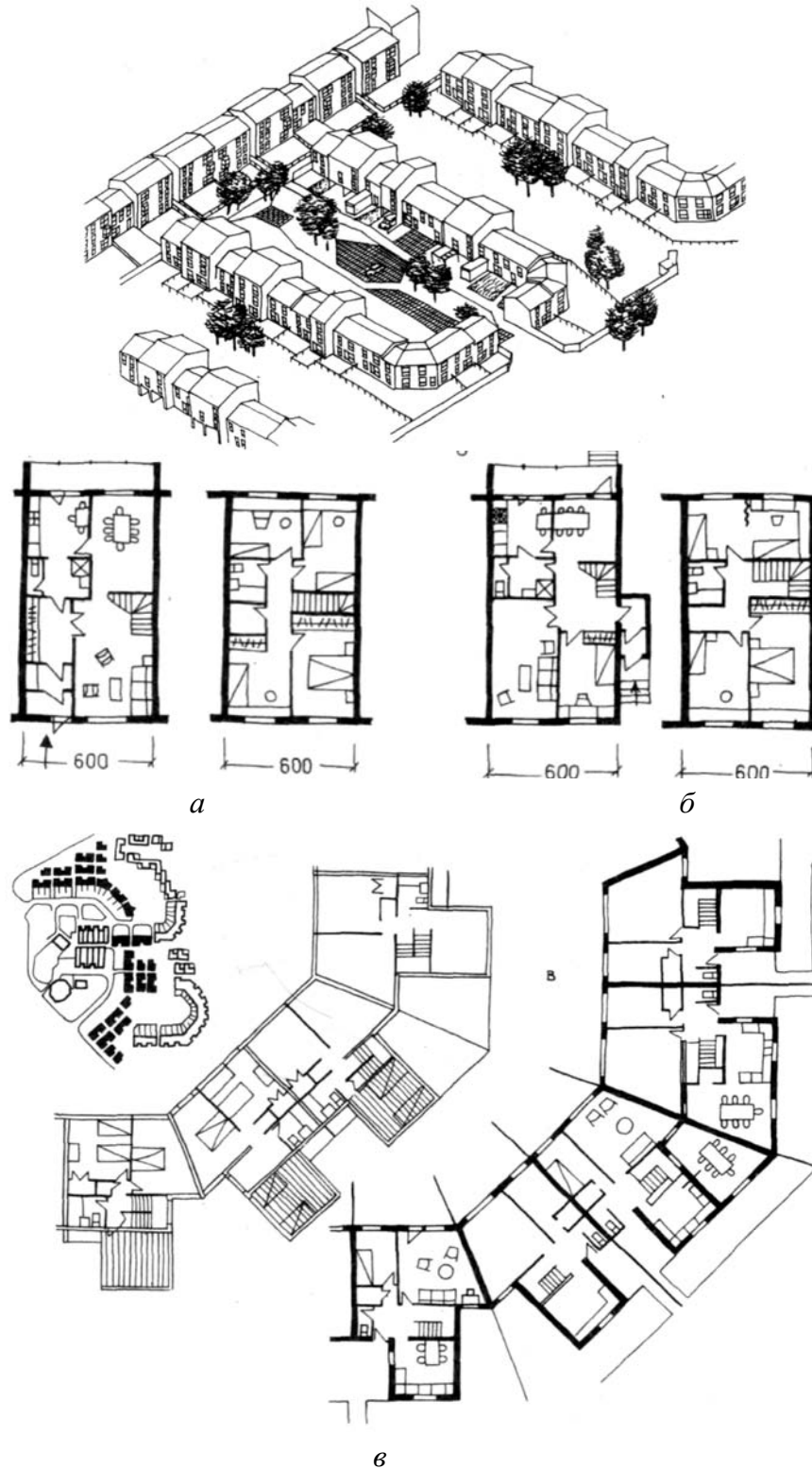
Рис. 27. Поселок в пригороде Лондона. Типы блоков: a — рядовой; б — торцевой; в — поворотный. Общий вид, планы первого и второго этажей, генеральный план
