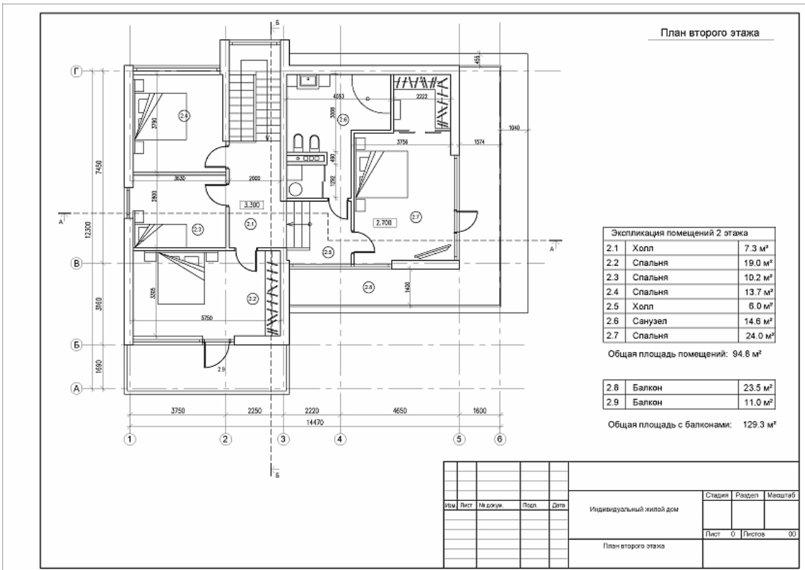
Рис. П.12. Планы этажей жилого дома. Вариант «Б»
