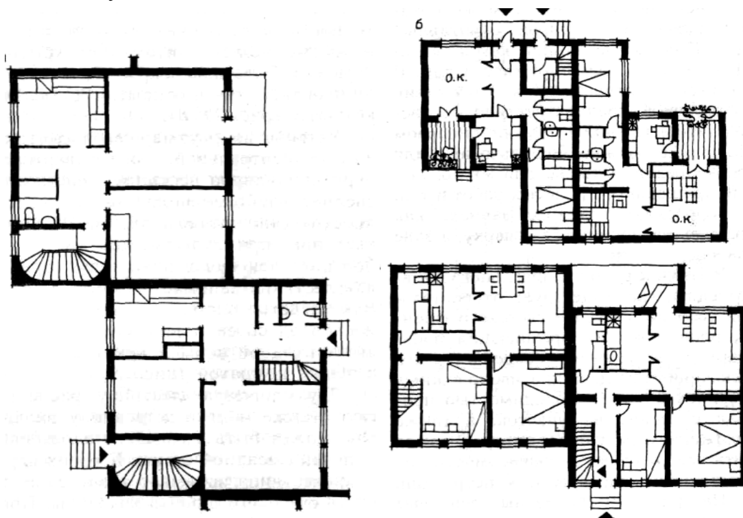
Рис. 32. Двухквартирные блоки с поэтажным расположением квартир: слева — при входах с разных сторон; справа сверху — при отдельных входах с одной стороны дома; справа внизу — с общим входом в верхние и нижние квартиры
