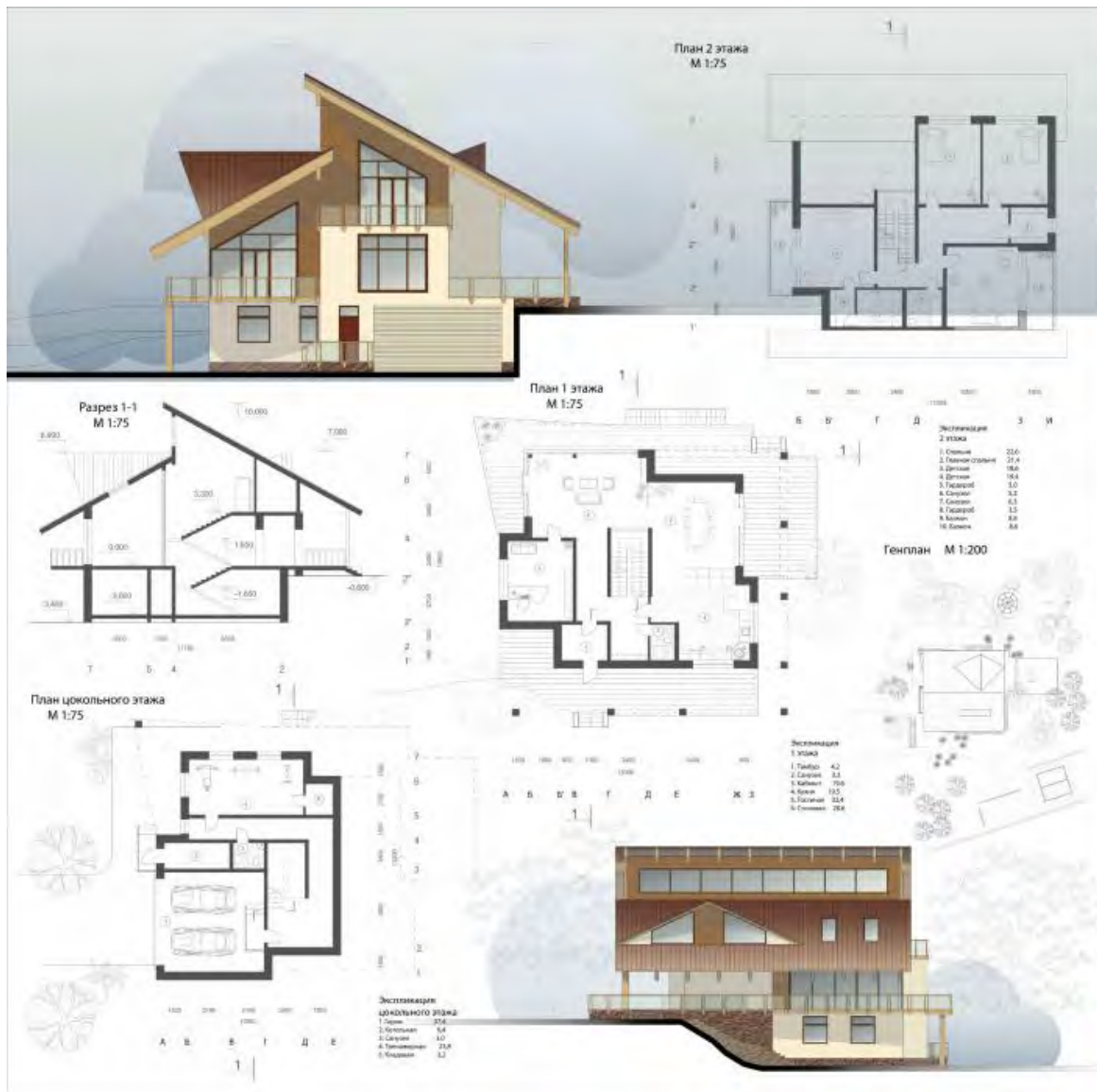
Рис. П.64. Малоэтажный индивидуальный жилой дом. Студ. Работа
