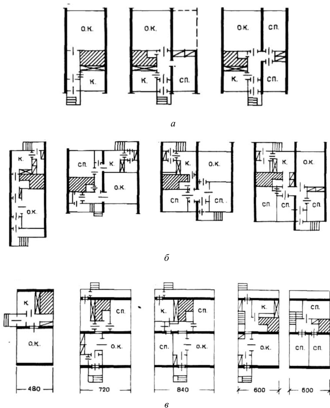
Рис. 25. Планировочные схемы серий блок - квартира: а — с продольными несущими стенами; б, в. — с поперечными несущими стенами
