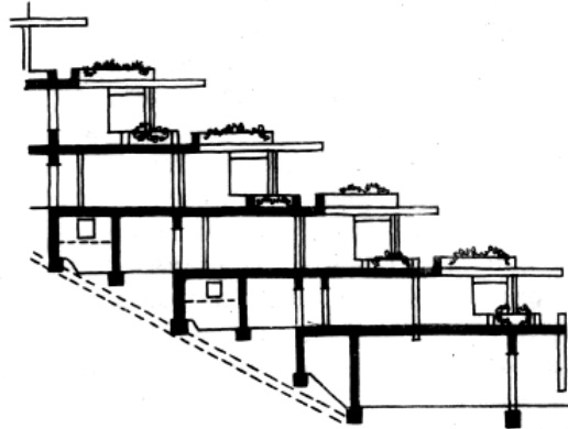
Рис. 50. Террасный жилой дом на рельефе: a — фрагмент застройки; б — Г-образная в плане блок-квартира; в — разрез по склону
