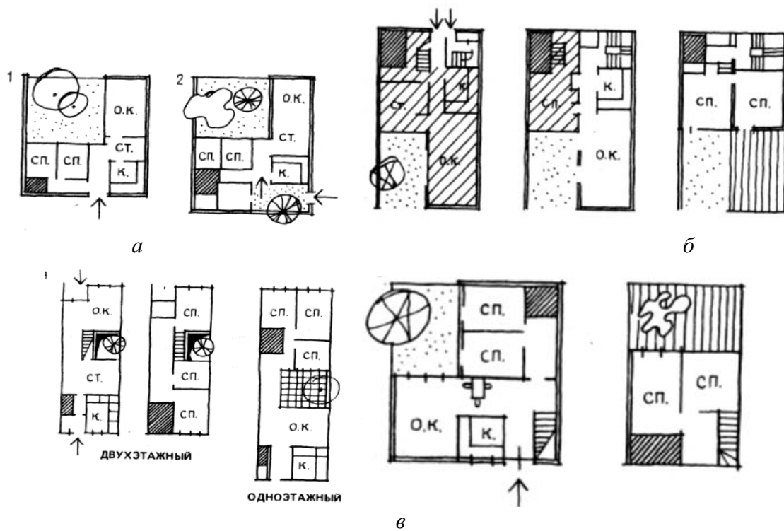
Рис. 47. Схемы блок-квартир с двориками: а — рядовые атриумные блок-квартиры; б — Г-образные блок-квартиры: 1 — с одним двориком; 2 — с двумя двориками; 3 — с частичным вторым этажом; в — Г-образная блок-квартира с поэтажным расположением квартир
