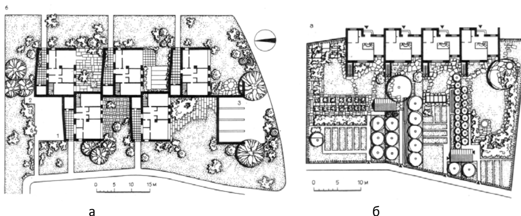
Рис. 5. Примеры решения участков блокированных домов разной площади: а — четырехквартирный дом с участками 600, 300, 350 и 500 \text{ м}^2 (дома для шахтеров, Англия); б — пятиквартирный блокированный дом с участками 150 — 200 \text{ м}^2 (ФРГ): 1 — площадка для игр детей; 2 — площадка для чистки одежды; 3 — индивидуальные гаражи
