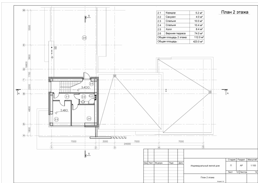
Рис. П.23. Планы этажей двухэтажного жилого дома. Вариант «Г»
