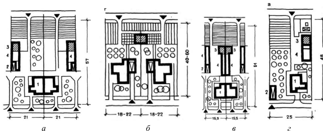
Рис. 2. Планировка участка приусадебных домов с отдельно стоящими хозяйственными постройками: а — хозяйственные помещения (кроме гаража) сгруппированы в одной постройке; б — хозяйственные помещения с гаражом; в — хозяйственные помещения в двух постройках; г — хозяйственные помещения частично пристроены к дому, частично вынесены в глубину участка: 1 — жилой дом; 2 — гараж; 3 — помещения для домашних или декоративных животных и птицы; 4 — хозяйственные помещения
