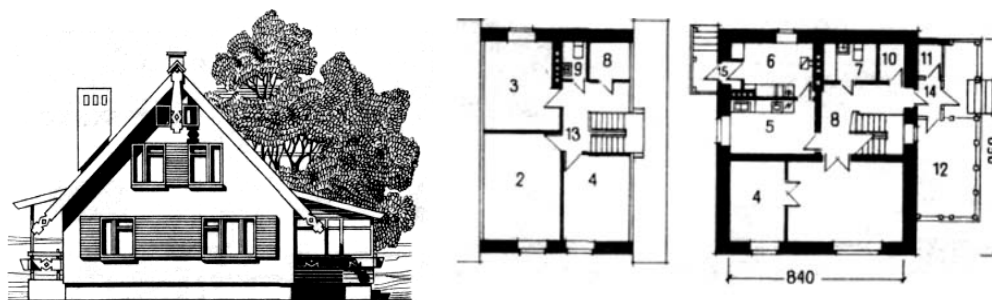
Рис. 18. Мансардный одноквартирный пятикомнатный жилой дом. Типовой проект. Фасад, план мансарды, план первого этажа: 1— общая комната; 2—4 — спальные комнаты; 5 — кухня; 6 — рабочая комната; 7 — санузел; 8 — прихожая; 9 — туалет; 10, 11— хозяйственная кладовая и шкафы; 12 — веранда; 13 — коридоры; 14, 15 — тамбуры
