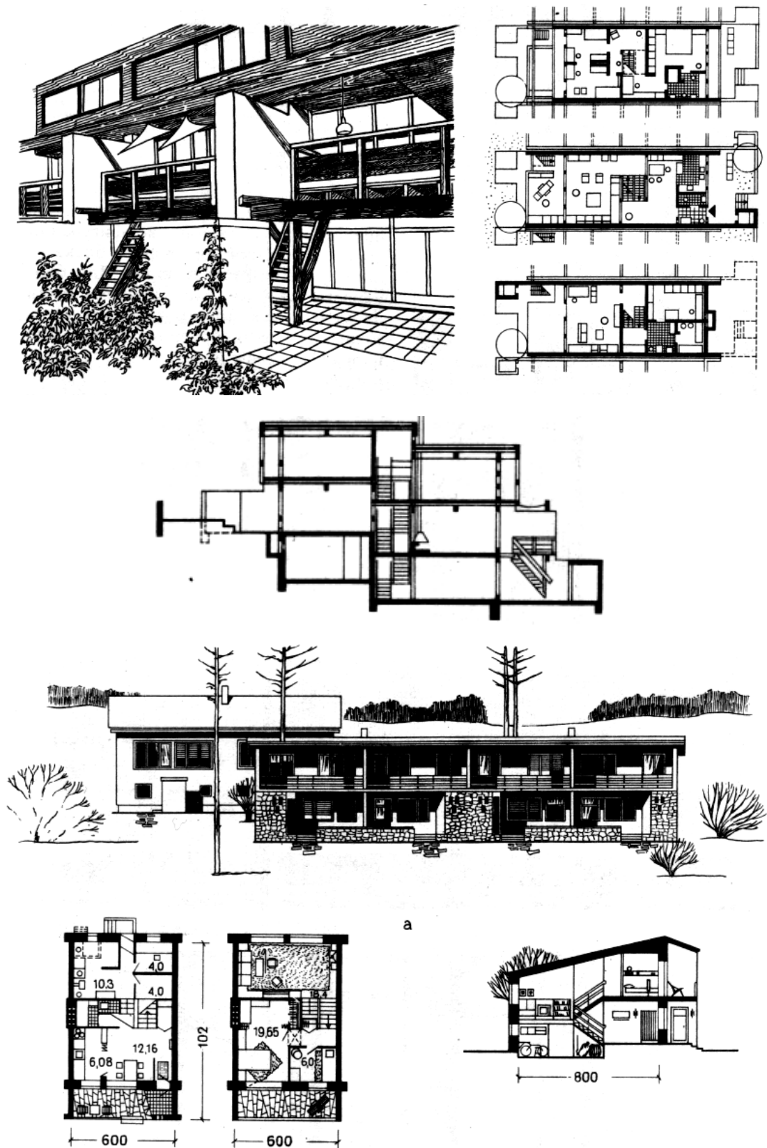
Рис. 40. Блокированные дома с квартирами, решенными со смещением уровней помещений на пол-этажа. Общий вид зданий, планы этажей, разрезы: а — застройка на склоне; б — застройка на ровном участке
