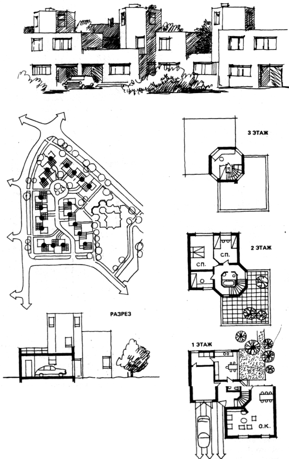
Рис. 43. Застройка трехэтажными жилыми блоками сложной объема и конфигурации
