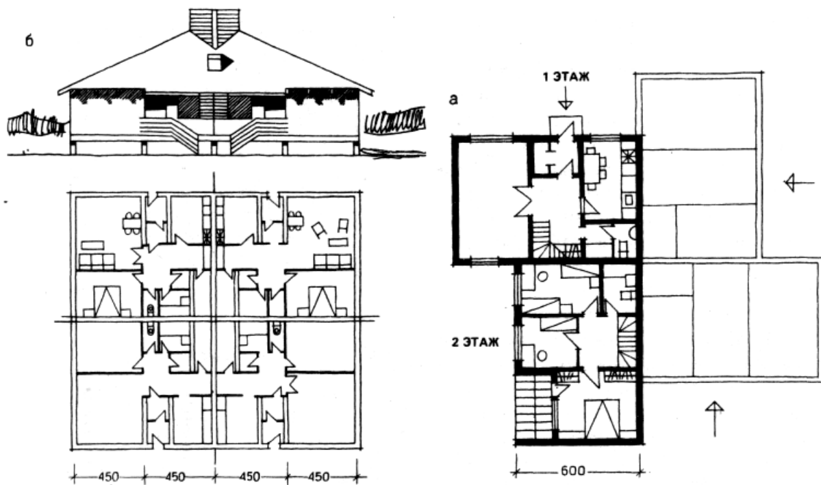
Рис. 46. Крестообразные блоки: слева — четырехквартирный одноэтажный блок-дом с двухкомнатными квартирами для крайнего севера; справа — двухэтажный блок-дом с четырехкомнатными квартирами
