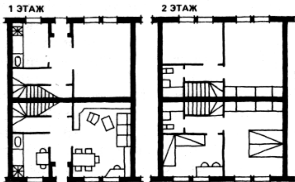
Рис. 45. Двухквартирный блок с трехкомнатными квартирами, все квартиры с односторонней ориентацией
