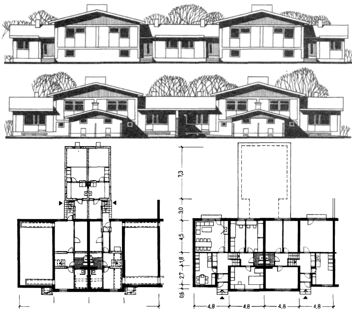
Рис. 30. Двухквартирный блок с четырехкомнатными квартирами в двух уровнях (с перепадом на пол-этажа) и цокольным этажом (Россия). Фасады, планы
