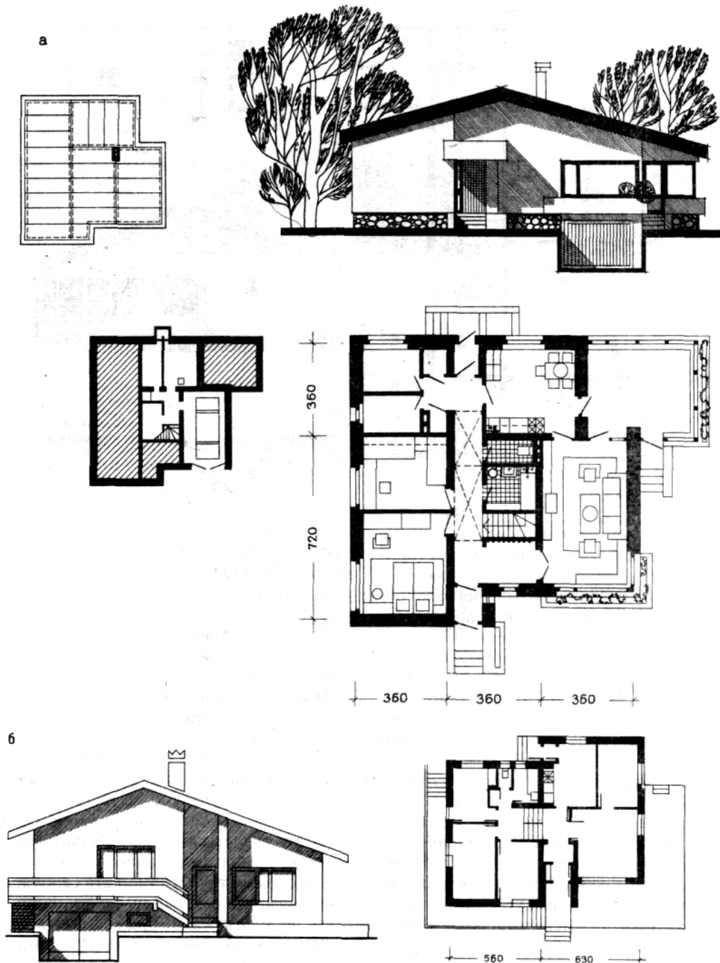
Рис. 13. Трехкомнатный дом с входом с угла и расположением хозяйственной зоны с боковой стороны дома. План этажа, схемы двухкомнатного и четырехкомнатного домов (вверху справа), фасад
