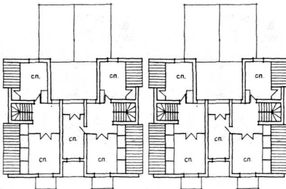
Рис. 24. Планы второго и первого этажей мансардного двухквартирного дома с трех- и пятикомнатными квартирами (МАРХИ)
