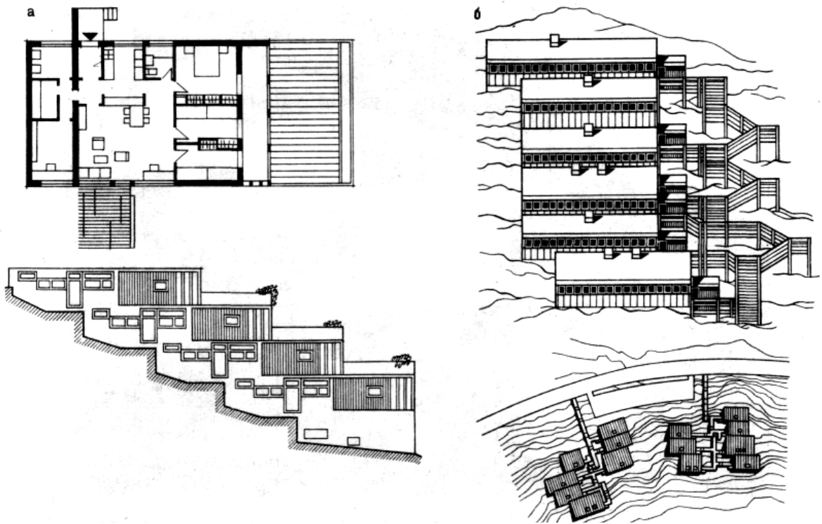
Рис. 51. Террасные блокированные дома на участках с сильным рельефом: слева — жилой дом с блоками прямоугольной формы, расположенными поперек рельефа (Швейцария); справа — жилые дома с прямоугольными одно-, двухэтажными блоками, расположенными вдоль рельефа (Гренландия)
