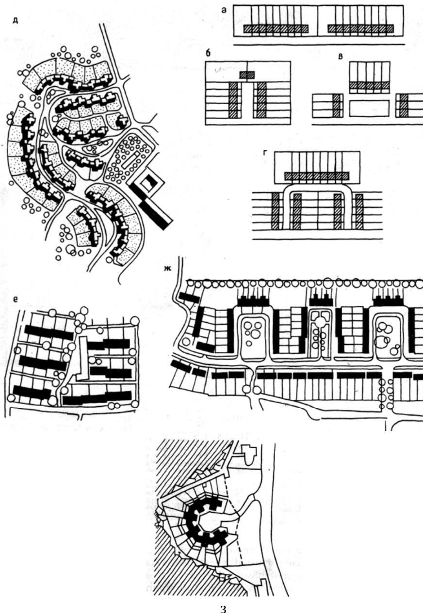
Рис. 56. Приемы застройки блокированными домами. Схемы застройки улиц: а — однорядная; б — тупиковая; в — с курдонерами; г — с петлеобразным проездом. Примеры застройки: д — фрагмент планировки и застройки совхоза «Агротехника» Ленинградской обл.; е — строчная застройка (ФРГ); ж — сочетание рядовой застройки с курдонерами (жилой комплекс, Англия); з — групповая застройка (жилой комплекс, Италия)
