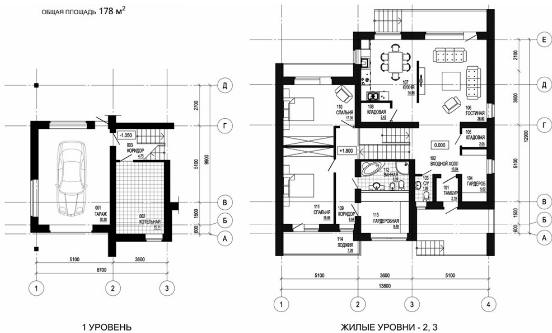
Рис. П.52. Планы двухэтажного жилого дома, общей площадью 178 м. кв.. Вариант «Р».
