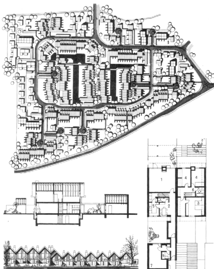
Рис. 39. Блокированные дома с входами в квартиры через хозяйственные постройки (жилой комплекс, ФРГ). Общий вид, застройка, генеральный план, план, разрез: 1 — общая комната; 2 — столовая; 3 — кухня; 4 — спальни; 5-7 — хозяйственные помещения, санузлы
