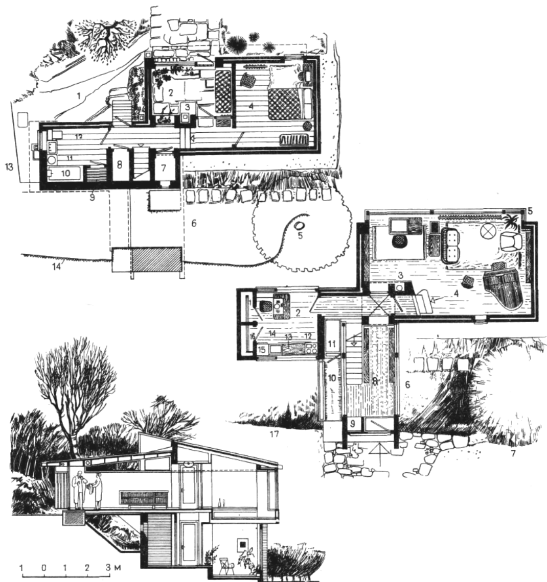
Рис. 21. Жилой одноквартирный дом на рельефе:
