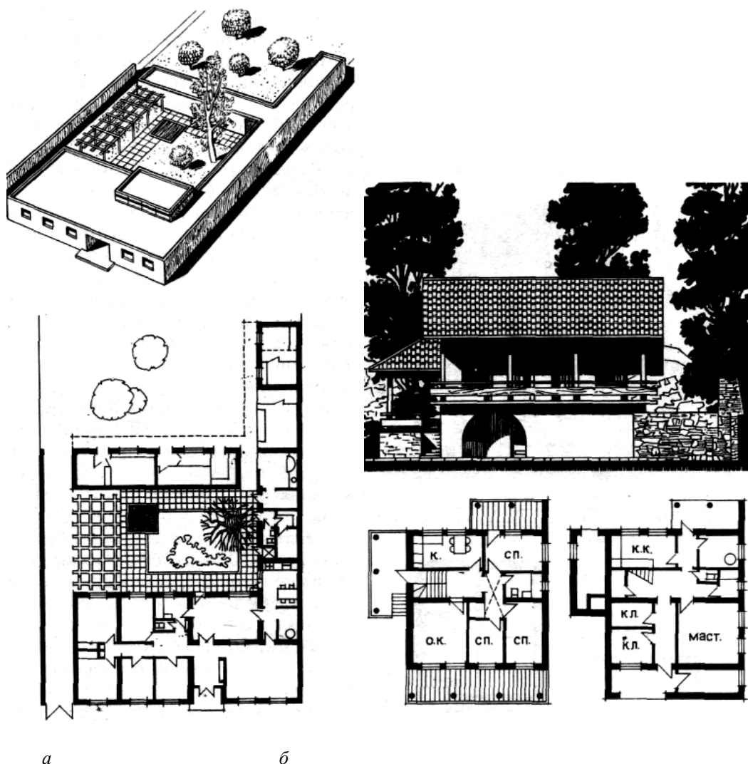
Рис. 11. Южный усадебный дом: а — жилой дом с развитым дворовым пространством для южных районов Средней Азии, общий вид, план этажа: б — двухэтажный дом для юга России, планы этажей, фасад
