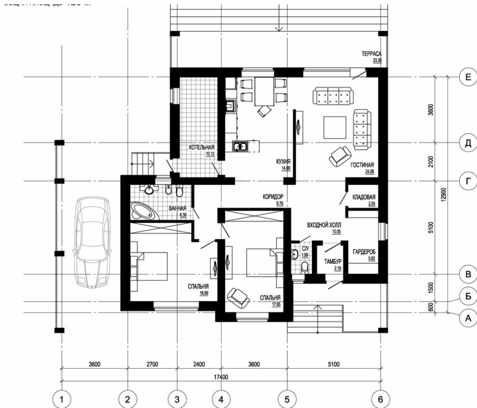
Рис. П.50. Общие виды и план одноэтажного жилого дома площадью 120 м. Вариант «П»
