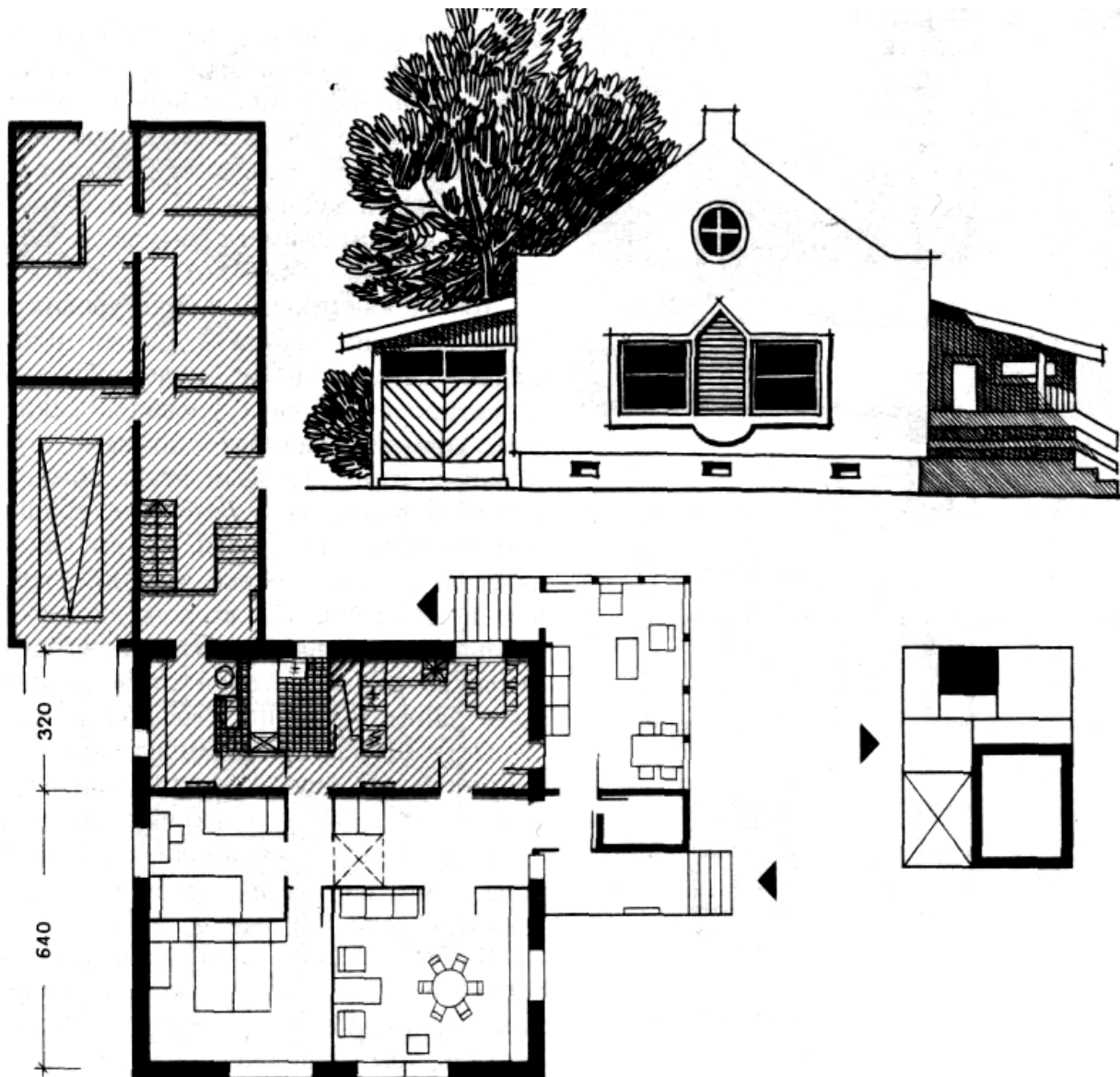
Рис. 12. Трехкомнатный жилой дом с входом с боковой стороны, хозяйственная зона с задней стороны дома. План этажа, схема двухэтажного дома, фасад
