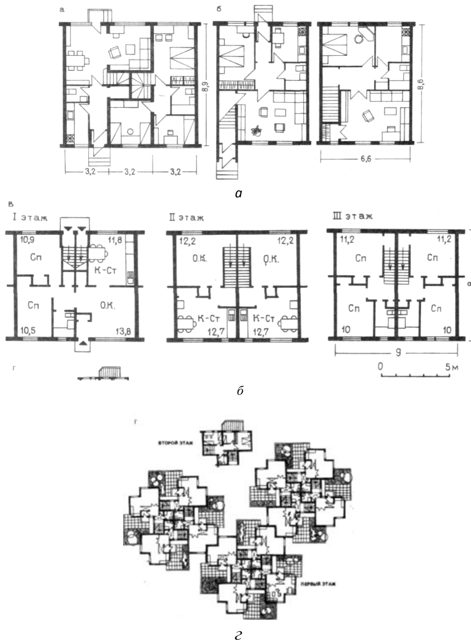
Рис. 29. Блоки с различным числом квартир: а — две двухэтажные квартиры в блоке; б — две поэтажные квартиры в блоке; в — три квартиры в блоке: одна в первом этаже, две двухэтажные над ней; г — четыре двухэтажные квартиры в блоке
