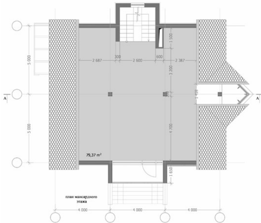
Рис. П.7. Планы этажей жилого дома. Вариант «А»
