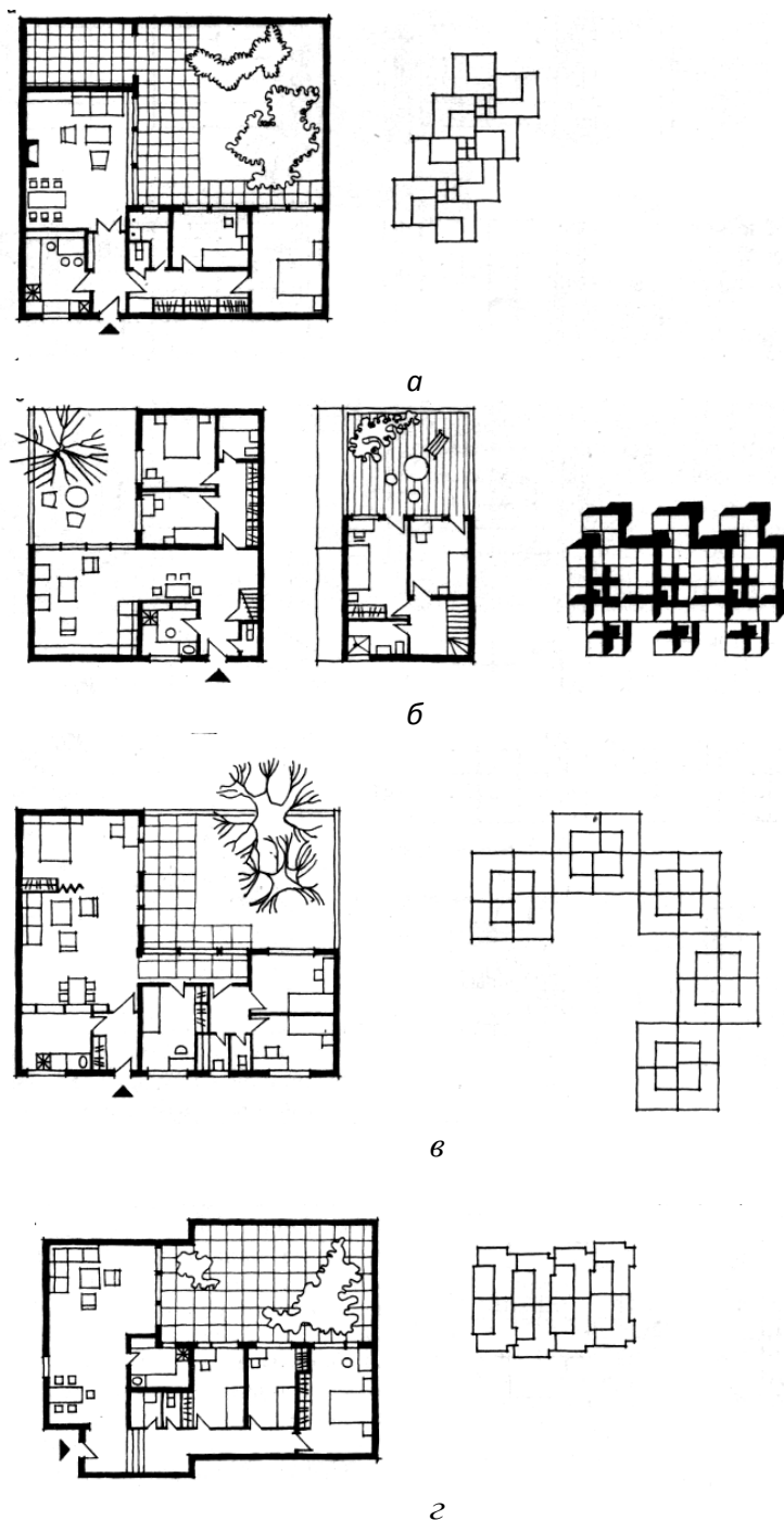
Рис. 48. Г-образные блок - квартиры с двориками: а — одноэтажный трехкомнатный блок; б — пятикомнатный блок с частичным вторым этажом; в — одноэтажный четырехкомнатный блок с коридором со стороны дворика; г — одноэтажный четырехкомнатный блок с кухней у внутреннего угла
