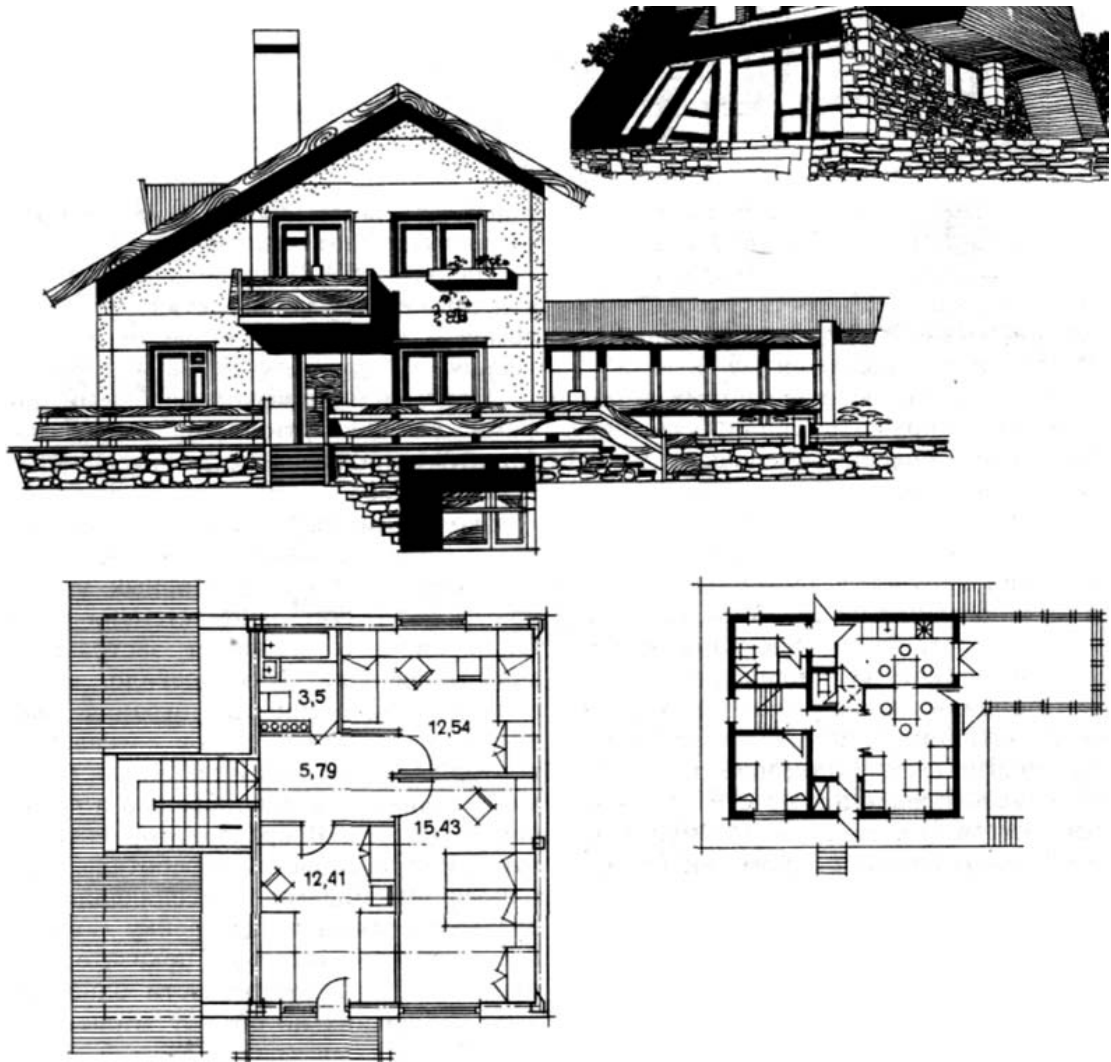
Рис. 20. Пятикомнатный двухэтажный дом с неполным верхним этажом. Фасад, план второго этажа (слева внизу), план первого этажа (справа)
