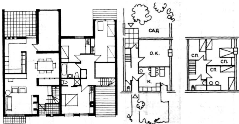
Рис. 26. Приемы планировки блок - квартир: а — общая комната расположена со стороны улицы, кухня — со стороны участка; б — кухня расположена со стороны улицы, общая комната — со стороны участка
