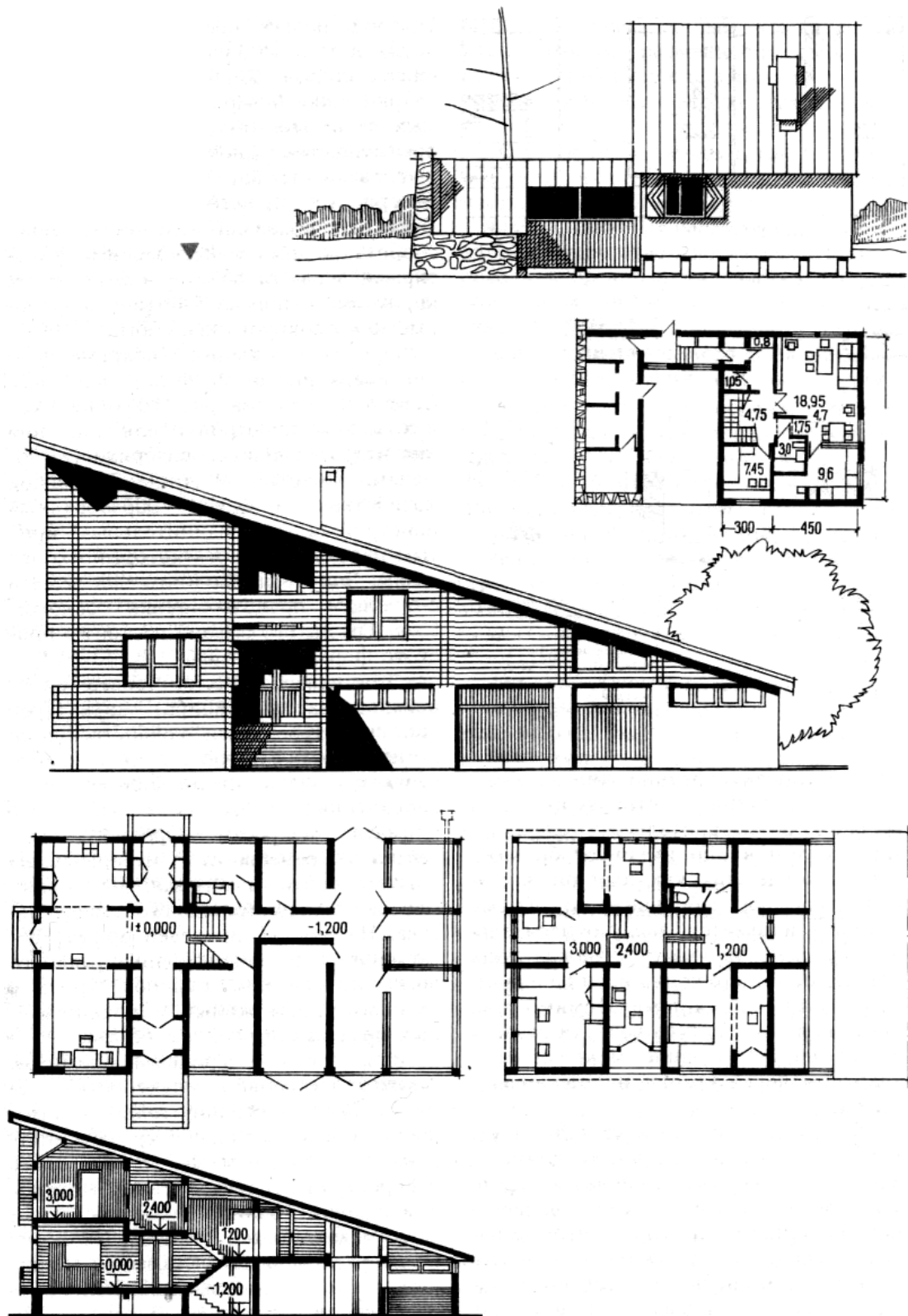
Рис. 8. Одноквартирный дом для Крайнего Севера. Типовой проект: фасад, план
