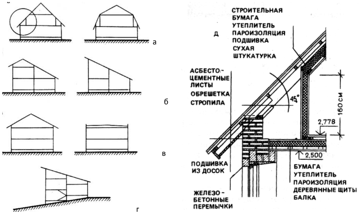
Рис. 17. Приемы решения жилых домов в двух уровнях: а — с мансардой без излома и с изломом крыши; б — часть квартиры расположена в двух уровнях (с чердаком или без чердака); в — вся квартира расположена в двух уровнях (с чердаком и без чердака); г — дом с перепадом уровней полов на пол-этажа; д — фрагмент разреза дома с мансардой
