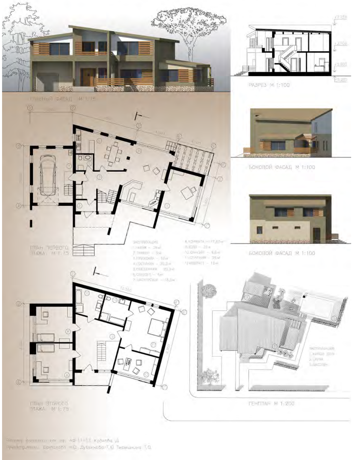
Рис. П.68. Малоэтажный индивидуальный жилой дом. Студ. Работа
