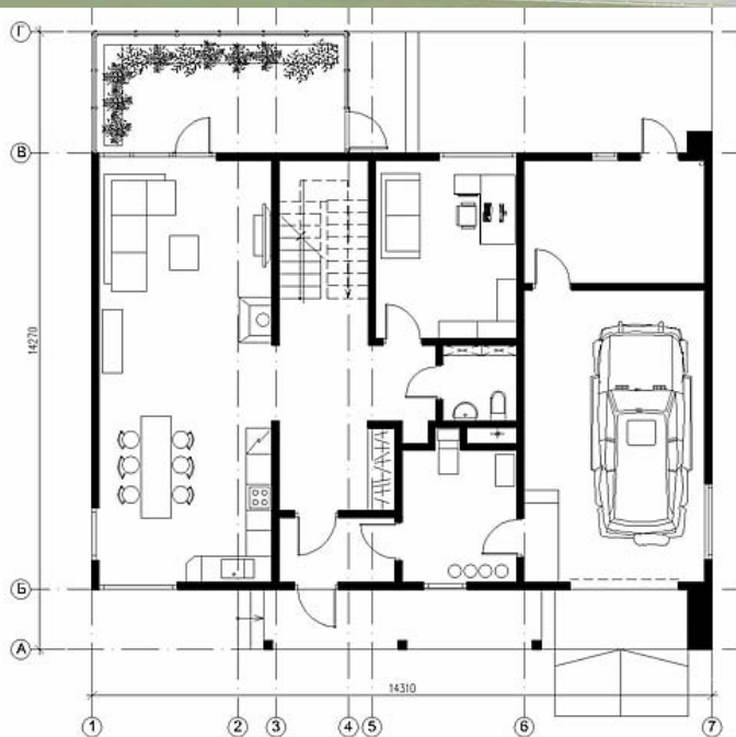
Рис. П.13. Общий вид и план 1-го этажа двухэтажного жилого дома. Вариант «В»
