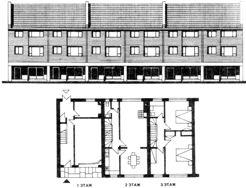
Рис. 41. Трехэтажный блокированный дом с расположением в первом этаже гаража и хозяйственных помещений, в верхних — жилых комнат (Англия)
