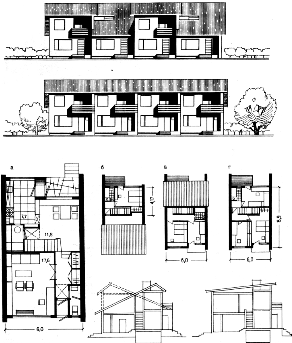
Рис. 35. Серия блок - квартир с поперечными несущими стенами (конкурсный проект): а — первый этаж, общий для всех блоков; б — двухкомнатная квартира; в — трехкомнатная квартира; г — четырехкомнатная квартира. Фасады, планы, разрезы
