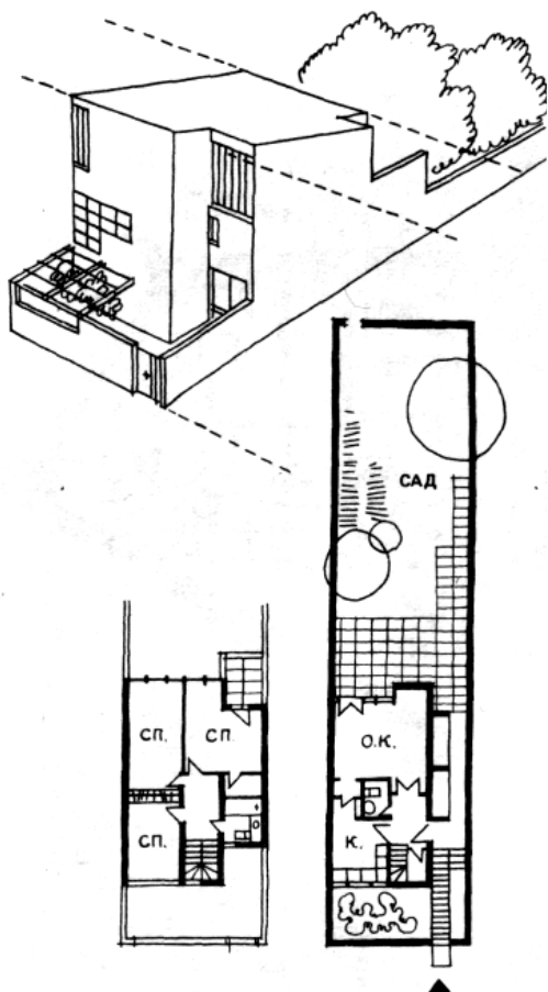
Рис. 38. Четырехкомнатная двухэтажная блок-квартира со сквозным проходом на участке вне дома. проходом на участке вне дома. Фасад, план
