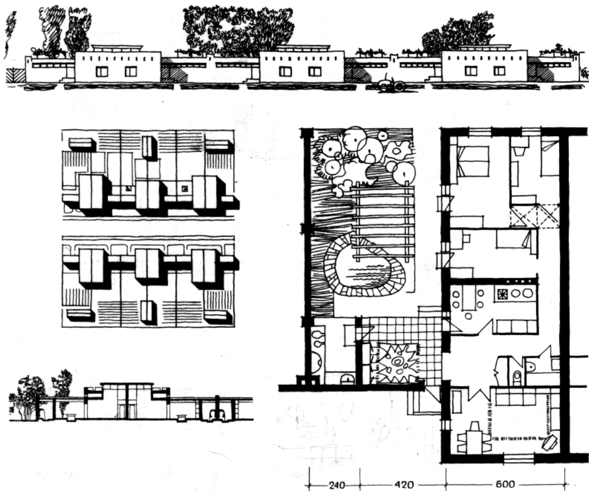
Рис. 58. Проект комплекса блокированных жилых домов для Средней Азии в условиях сейсмики. Конкурсный проект. Развертка по улице, фрагмент генерального плана, план блок - квартиры, разрез
