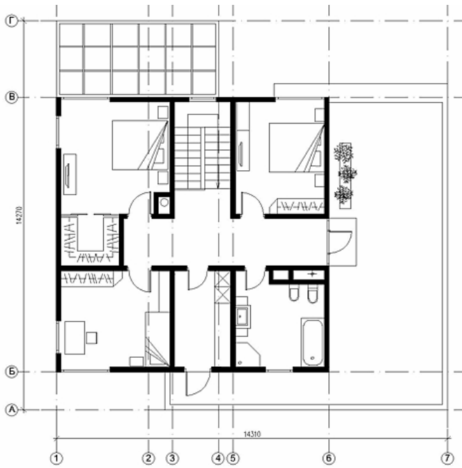
Рис. П.14. Общий вид и план 2-го этажа двухэтажного жилого дома. Вариант «В»
