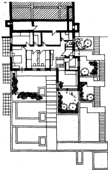
Рис. 50. Террасный жилой дом на рельефе: a — фрагмент застройки; б — Г-образная в плане блок-квартира; в — разрез по склону
