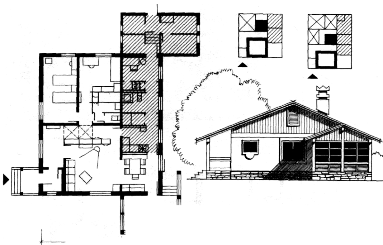
Рис. 14. Примеры домов с входами со стороны улицы, с расположением хозяйственной зоны с задней стороны дома: вверху — трехкомнатный дом; план перекрытия, план подвала, план первого этажа; внизу — четырехкомнатный дом фасад, план
