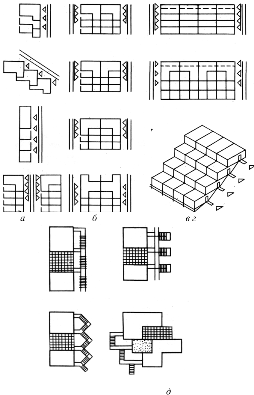
Рис. 49. Приемы блокировки и типы лестниц в террасных домах на рельефе: а — однорядная; б — двухрядная; в — многорядная; z — организация входов в квартиры при многорядной блокировке через поэтажные коридоры; д — типы лестниц в зависимости от уклона и приема блокировки
