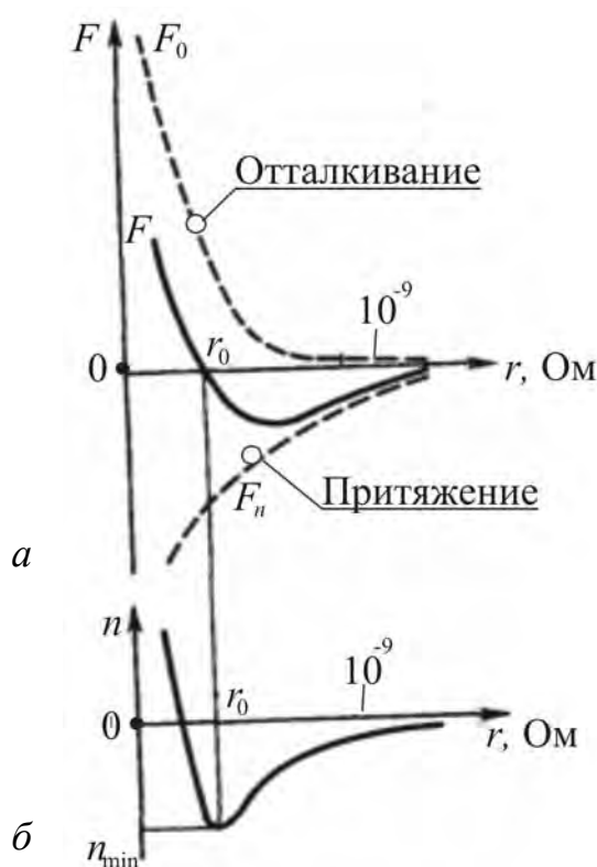
Рис. 3.2: а — силы, действующие на одну молекулу со стороны другой молекулы; б — график потенциальной энергии межмолекулярных взаимодействий
